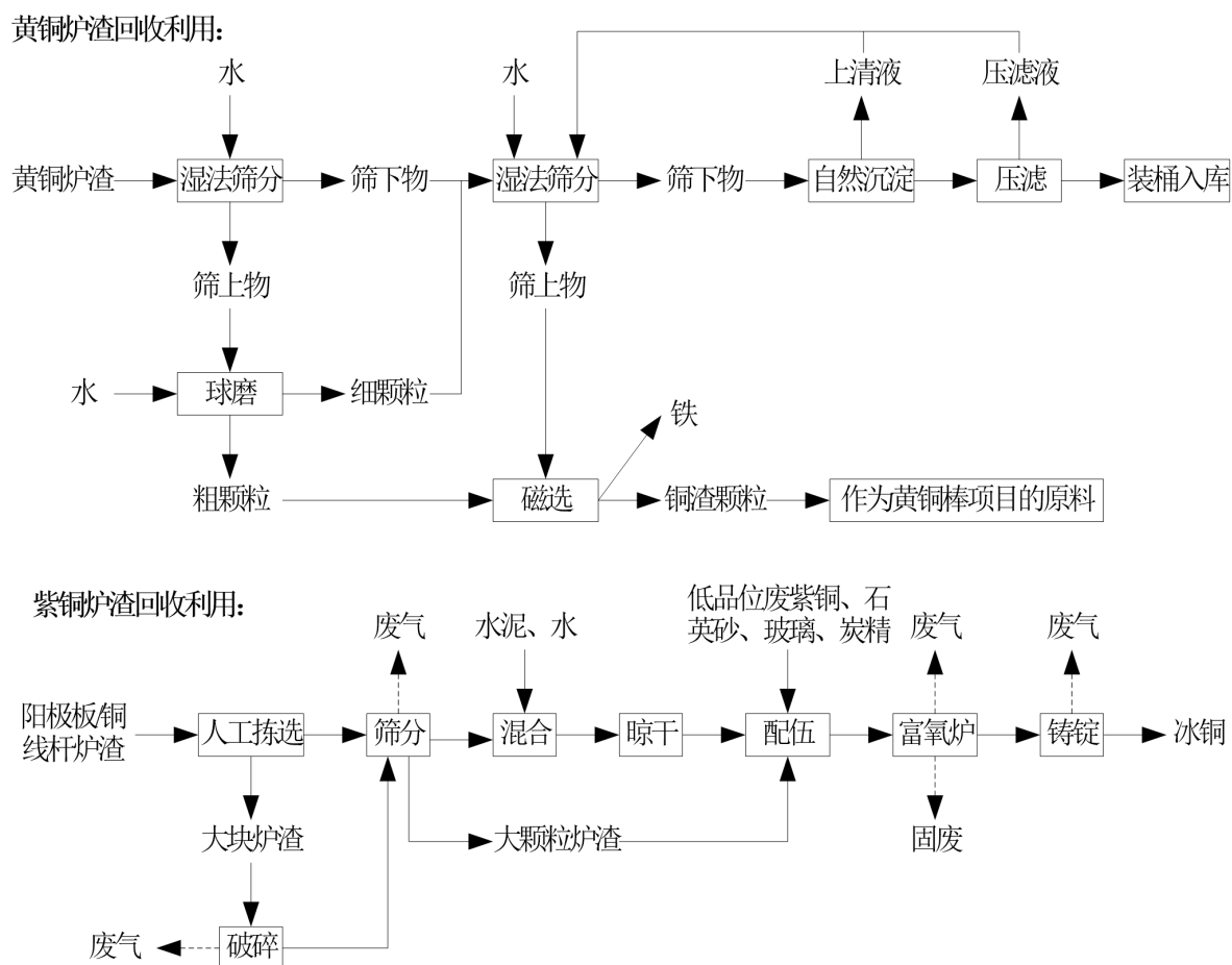
图 1-1 铜炉渣综合回收利用生产工艺流程图
